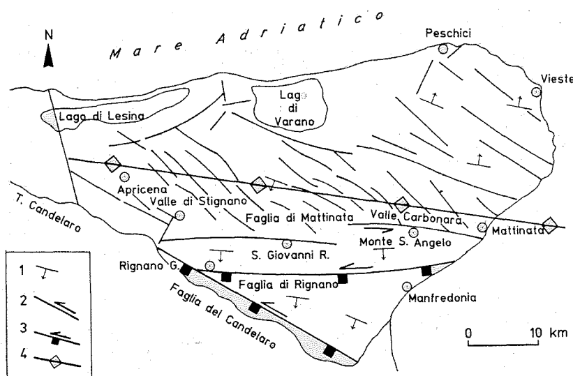
Fig.2 - Schema strutturale del Promontorio del Gargano (Billi e Salvini, 2000, modificato).
