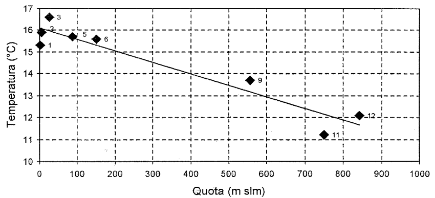
Fig. 7 - Retta di regressione quota-temperatura.
