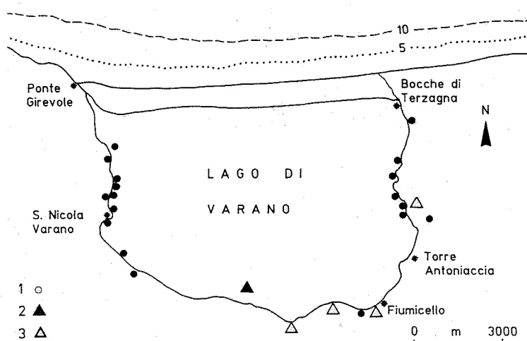
Fig.10: Schema degli efflussi individuati lungo le sponde del lago di Varano.
